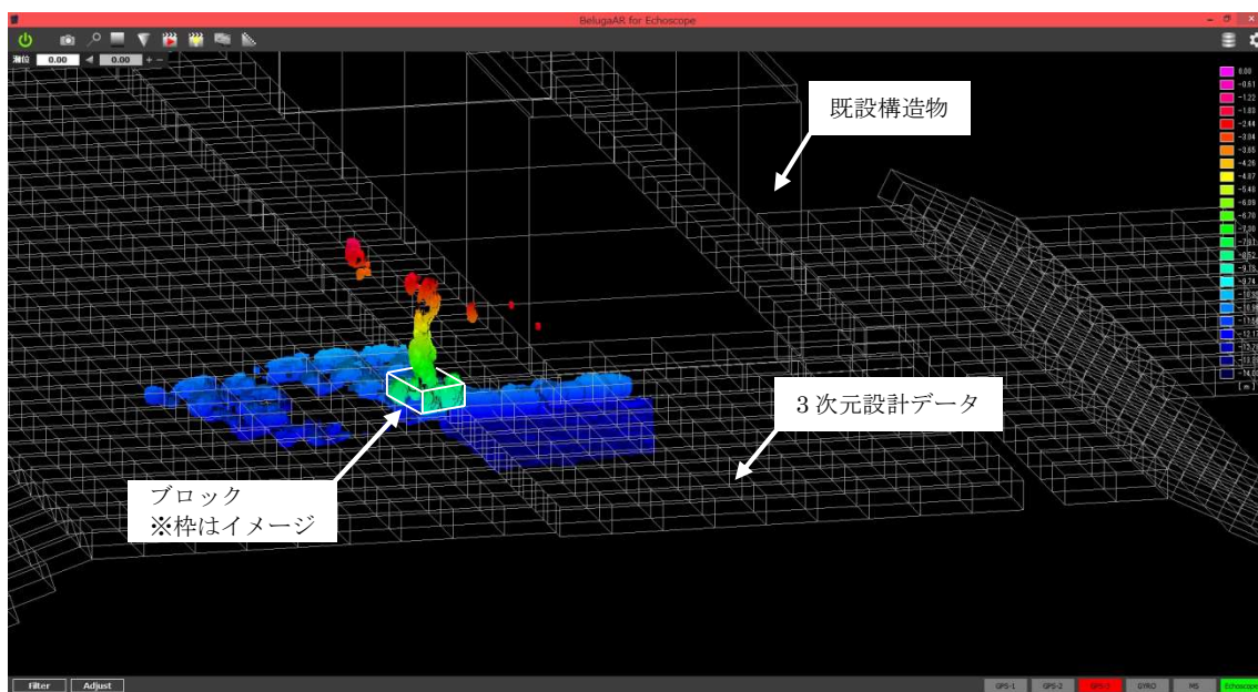
図3 ブロック据付状況（3次元水中ソナーによる施工管理）
