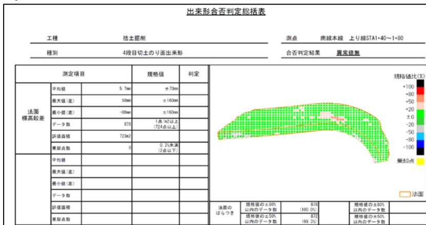
図. 2 ヒートマップによる出来形調査
