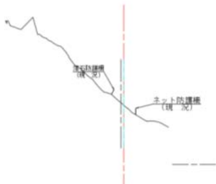
図 2 作成横断面図
