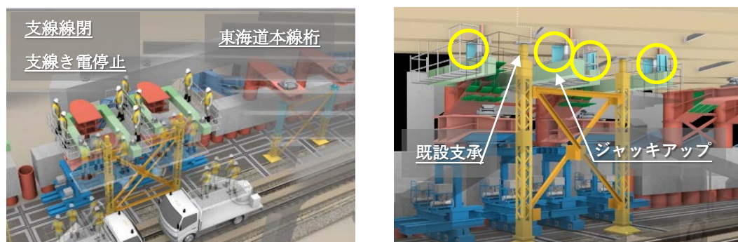
図-5 東海道本線桁の受替工事での活用
