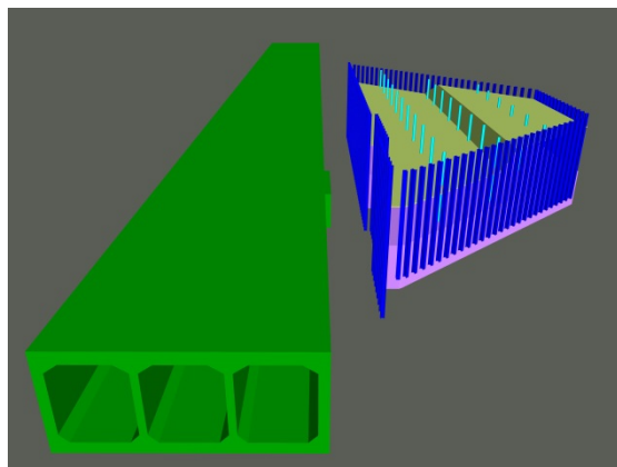
図-6 既設構造物と施工土留の3Dモデル
