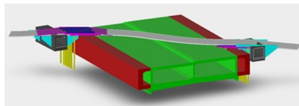
図-3 仮設計画
