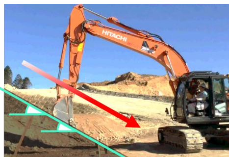
MCバックホウによる丁張レス施工 概念図
