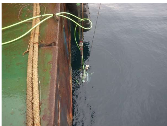
写真 4 水中ソナー設置状況
