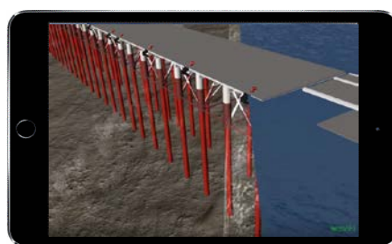
図-2 ARへの展開(画面ははめこみ合成)
