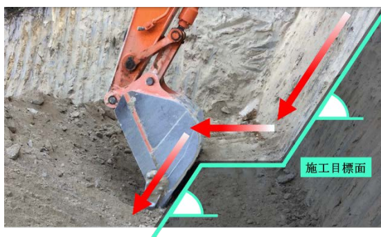
MCバックホウによる丁張レス施工 概念図
