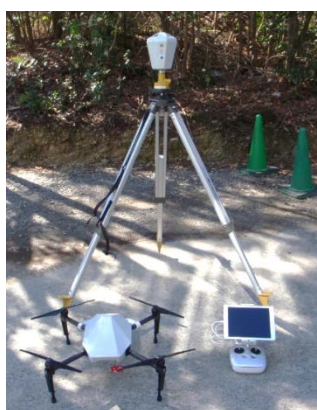
使用機材
