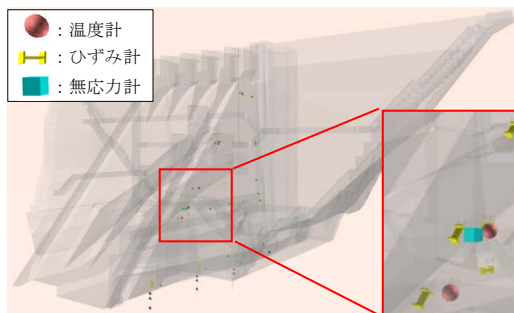
図-5 埋設工 3 次元モデル
