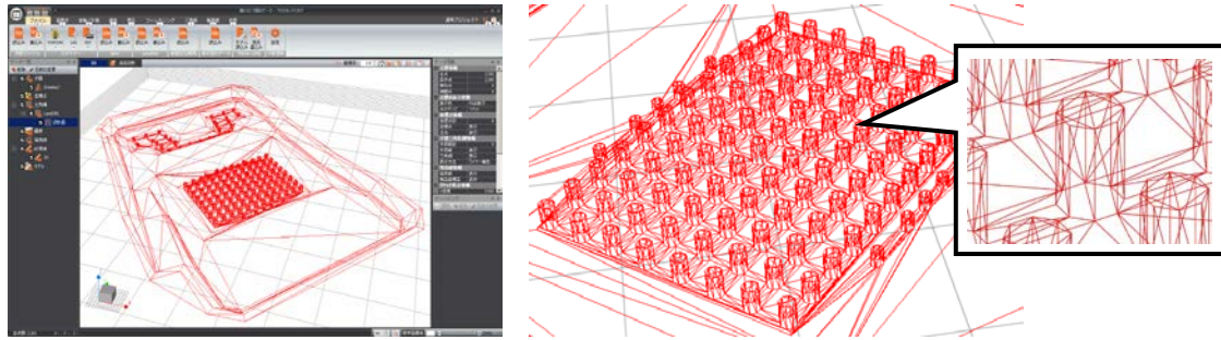
図-7 杭頭周囲の掘削用モデルを追加した ICT 建設機械用データ
