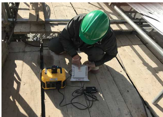
【屋内電波改善装置、ポータブル電源】
