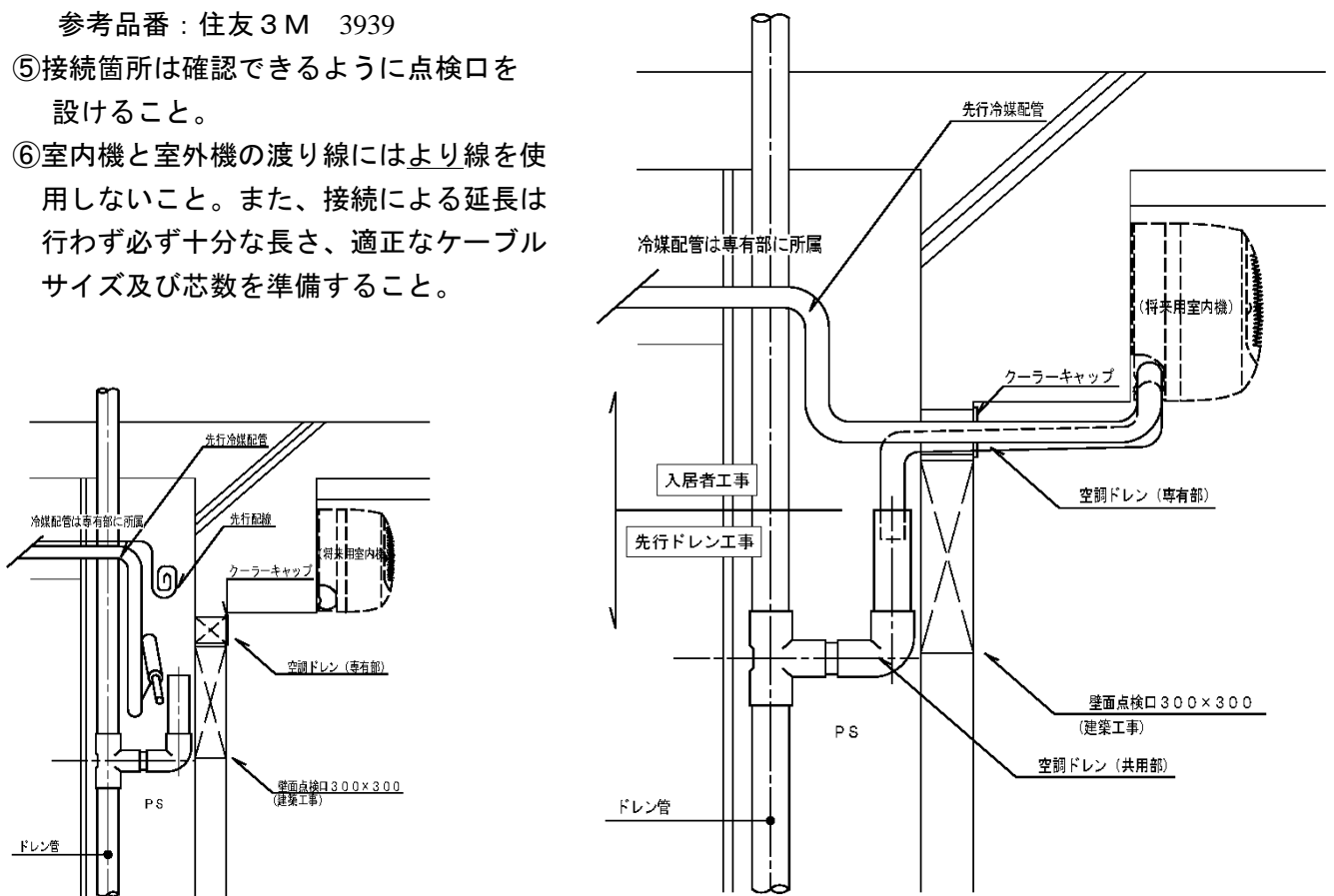
オプションエアコンドレン管 要領図
