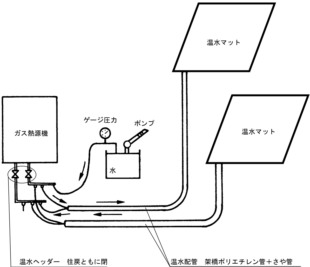
図-1 温水式床暖房のゲージ検査例
