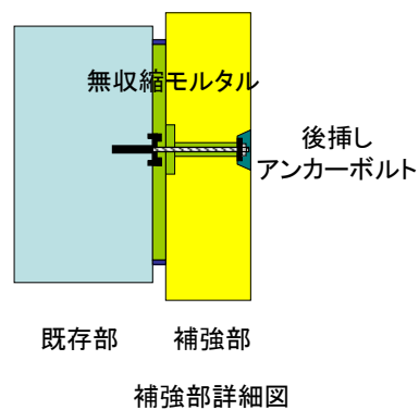
MaSTER FRAME構法の補強イメージ
