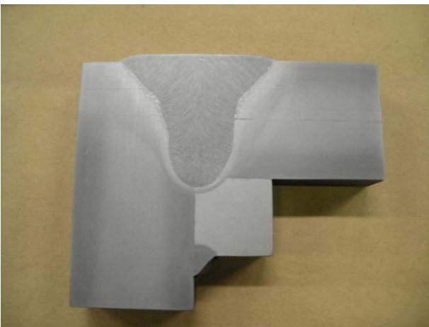
マクロ試験による、きずの有無や溶込みの確認
