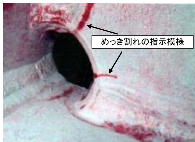
浸透探傷によるめっき割れの検査例 (通常は、目視検査で十分です)
