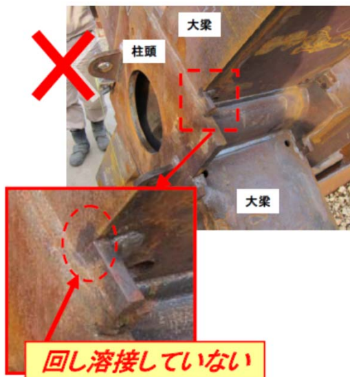
裏当て金のすき間
