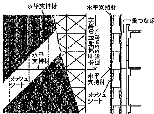
図 鋼管足場への設置例
