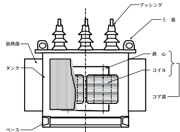
高圧変圧器の例
