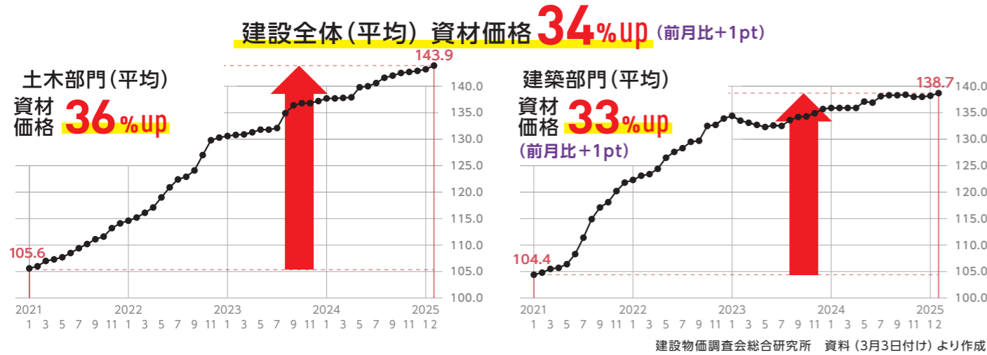
2021年1月～2025年2月の建設資材物価指数(東京)の推移 (2015年平均=100)
